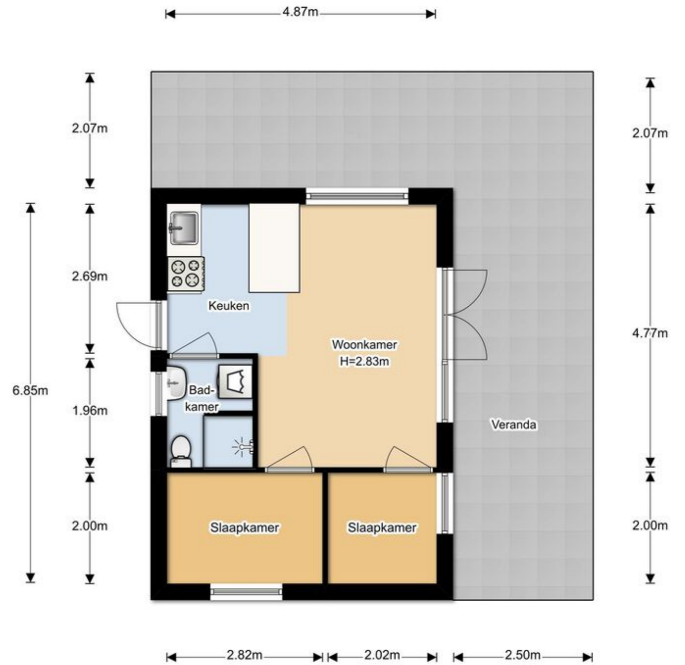
Begane Grond
